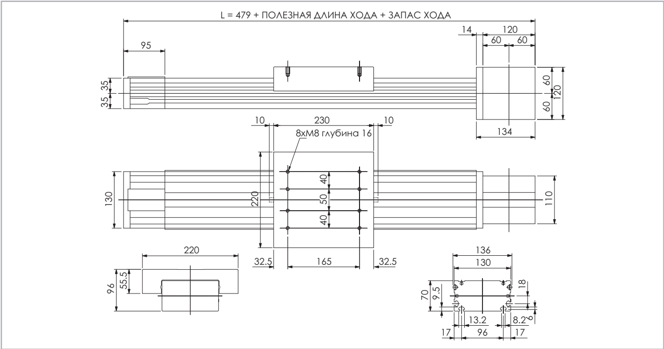
* Данные по величине запаса хода предоставляются под запрос, причём эта величина может быть различной, в зависимости от специфики решаемых Заказчиком задач. Рис. 30
