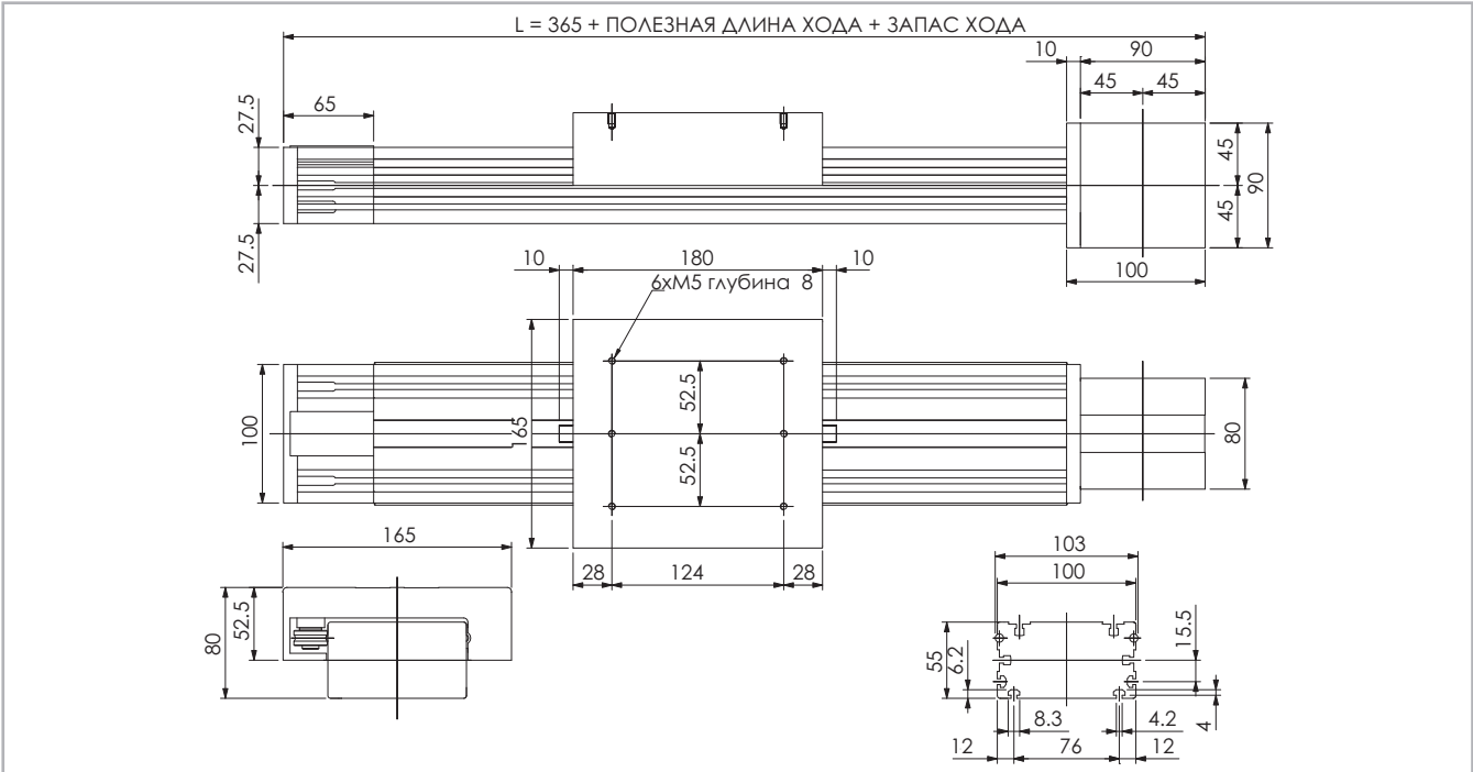
* Данные по величине запаса хода предоставляются под запрос, причём эта величина может быть различной, в зависимости от специфики решаемых Заказчиком задач. Рис. 26
